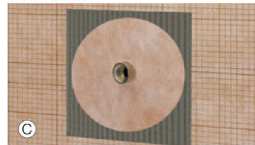
© Schlüter®-KERDI-KM (manžeta na potrubí) tloušťka = 0,1 mm
